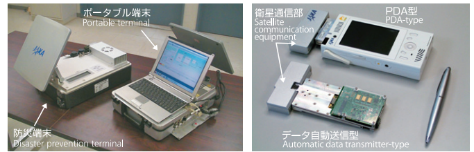
▲ 防災端末・ポータブル端末 Disaster prevention terminal/Portable terminal ▲ 超小型端末 Ultracompact terminal
